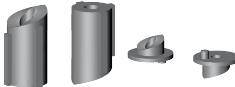
Steigeband Ober- und Unterteil Ø 21,5 mm, Steigung 5 mm auf 90° Fitting for increase, upper and lower part Ø 21.5 mm, pitch 5 mm on 90° Douille pour rehaussement, pièce supérieure et inférieure Ø 21,5 mm, montée 5 mm sur 90°
